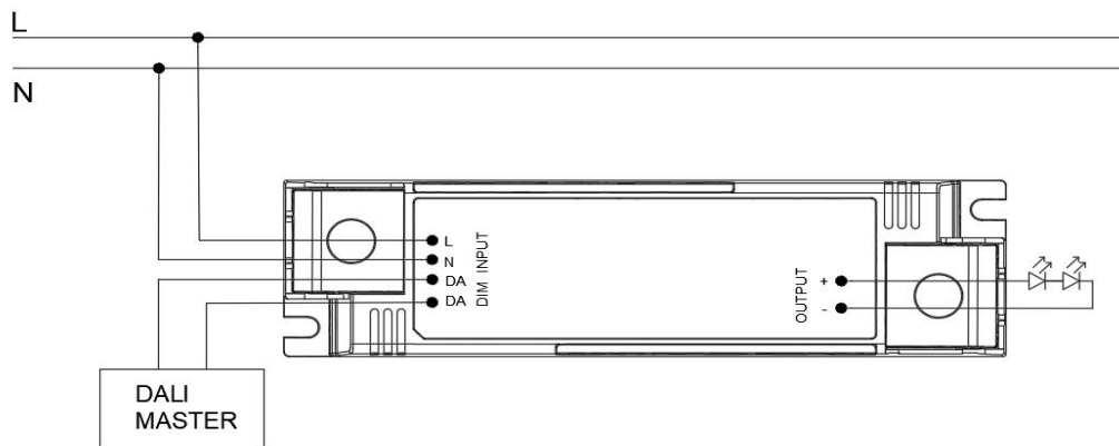
Fig. A: DALI Dimming
